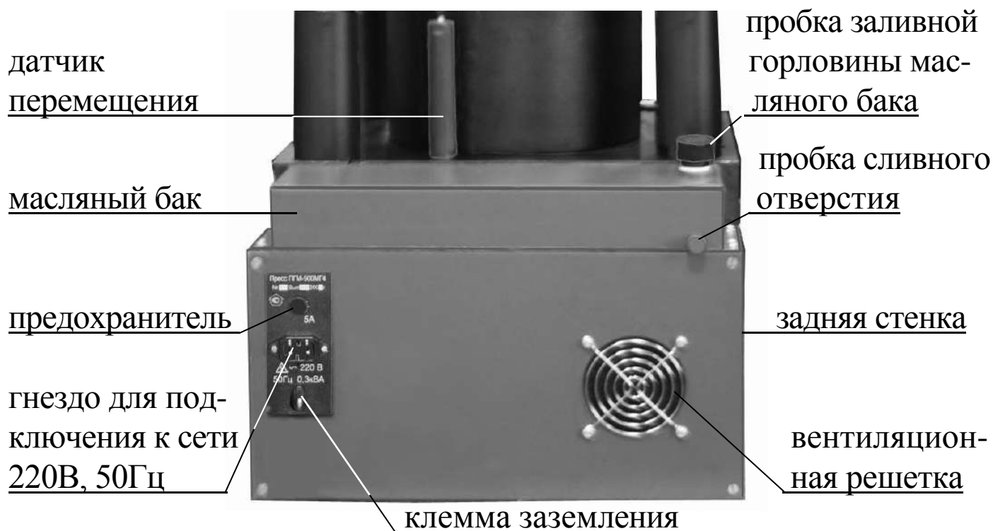
Рисунок 4.1.б – Внешний вид пресса. Вид сзади
